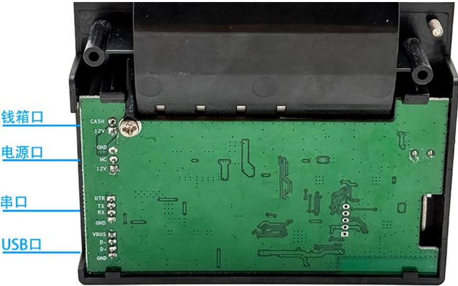
接口示意图
