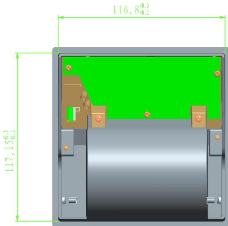
外形尺寸
