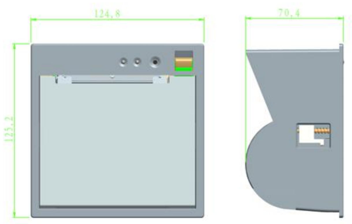
外形尺寸
